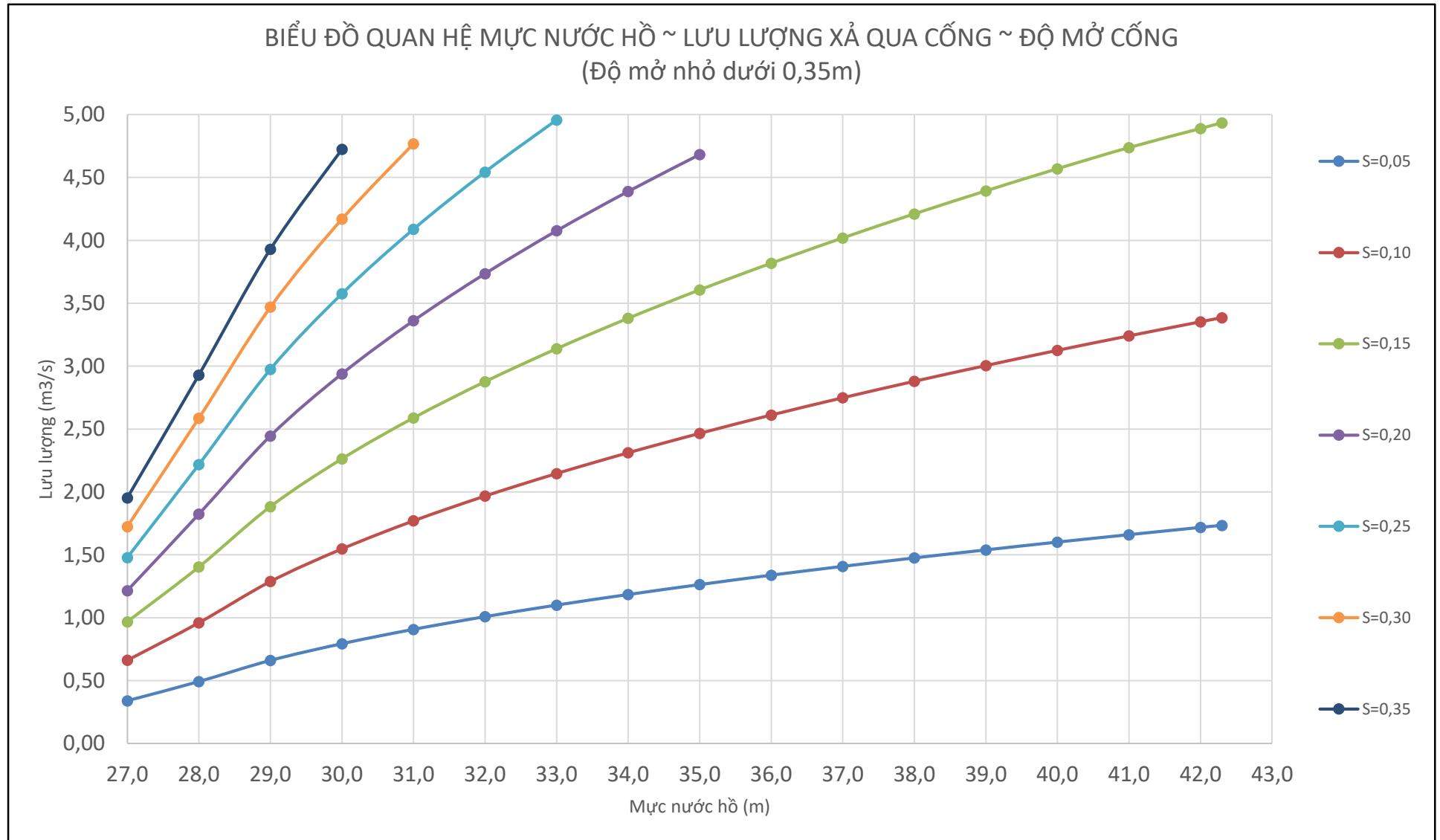
Hình PL 4.1: Hình vẽ quan hệ mực nước hồ ~ Q xả công ~ Độ mở cổng lấy nước
