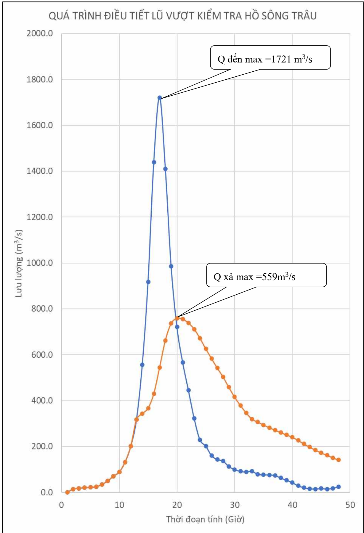
Hình PL 8.3: Quá trình điều tiết lũ vượt kiểm tra P=0,1%
