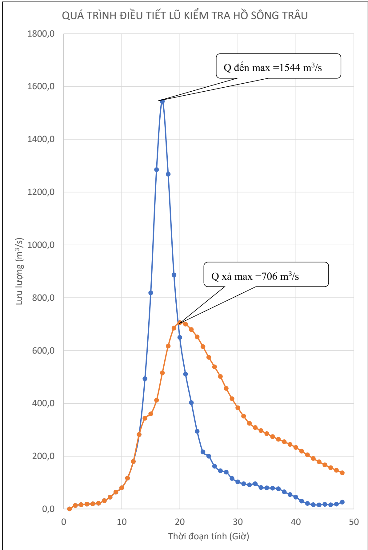
Hình PL 8.2: Quá trình điều tiết lũ kiểm tra P=0,2%
