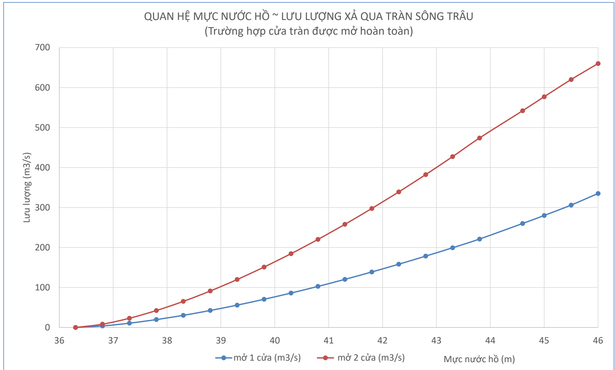
Hình PL 3.3: Lưu lượng qua tràn ~ Mức nước hồ ~ Độ mở cửa van (Trường hợp mở hoàn toàn)
