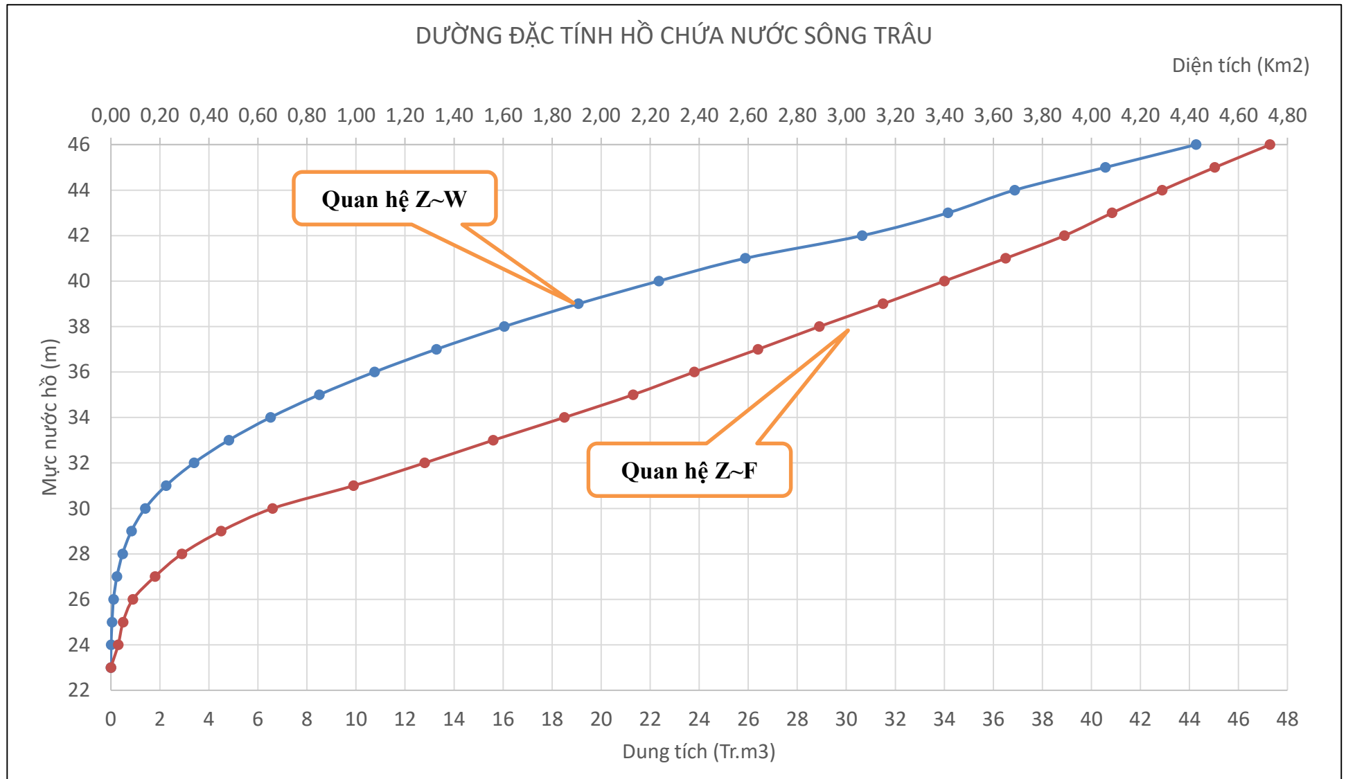
Hình PL2.1 Đường đặc tính hồ chứa nước Sông Trâu
