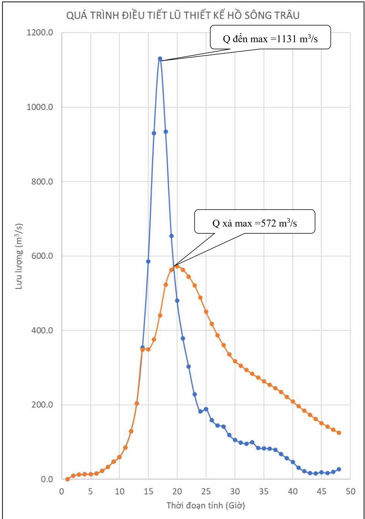
Hình PL 8.1: Quá trình điều tiết lũ thiết kế P=1,0%
