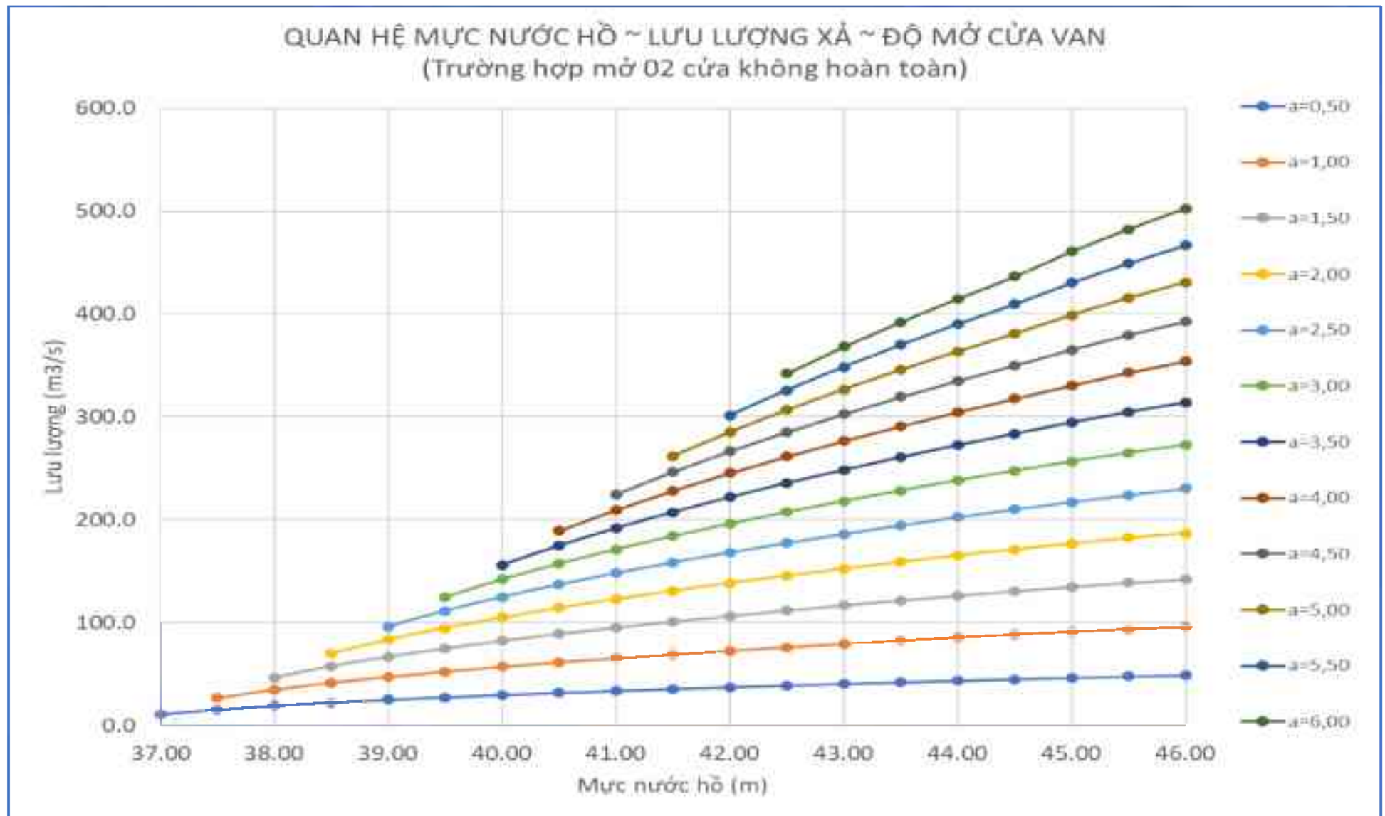
Hình PL 3.2: Lưu lượng qua tràn ~ Mức nước hồ ~ Độ mở cửa van (Trường hợp mở 2 cửa không hoàn toàn)
