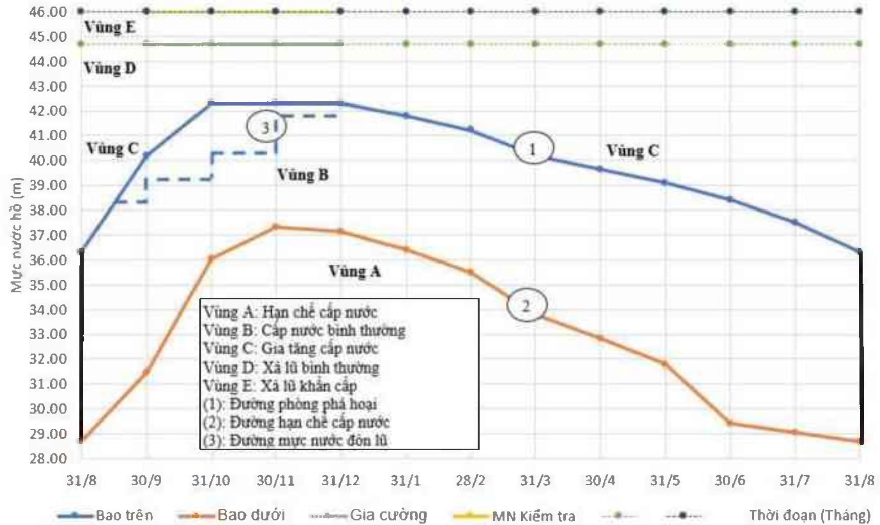
Hình PL5.1 Biểu đồ điều phối hồ chứa nước Sông Trâu
