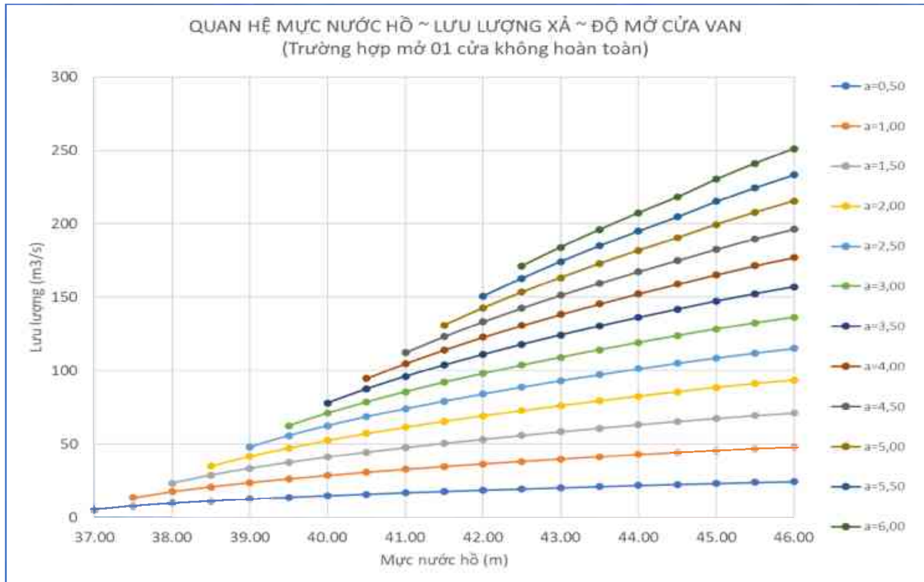
Hình PL 3.1: Lưu lượng qua tràn ~ Mức nước hồ ~ Độ mở cửa van (Trường hợp mở 1 cửa không hoàn toàn)
