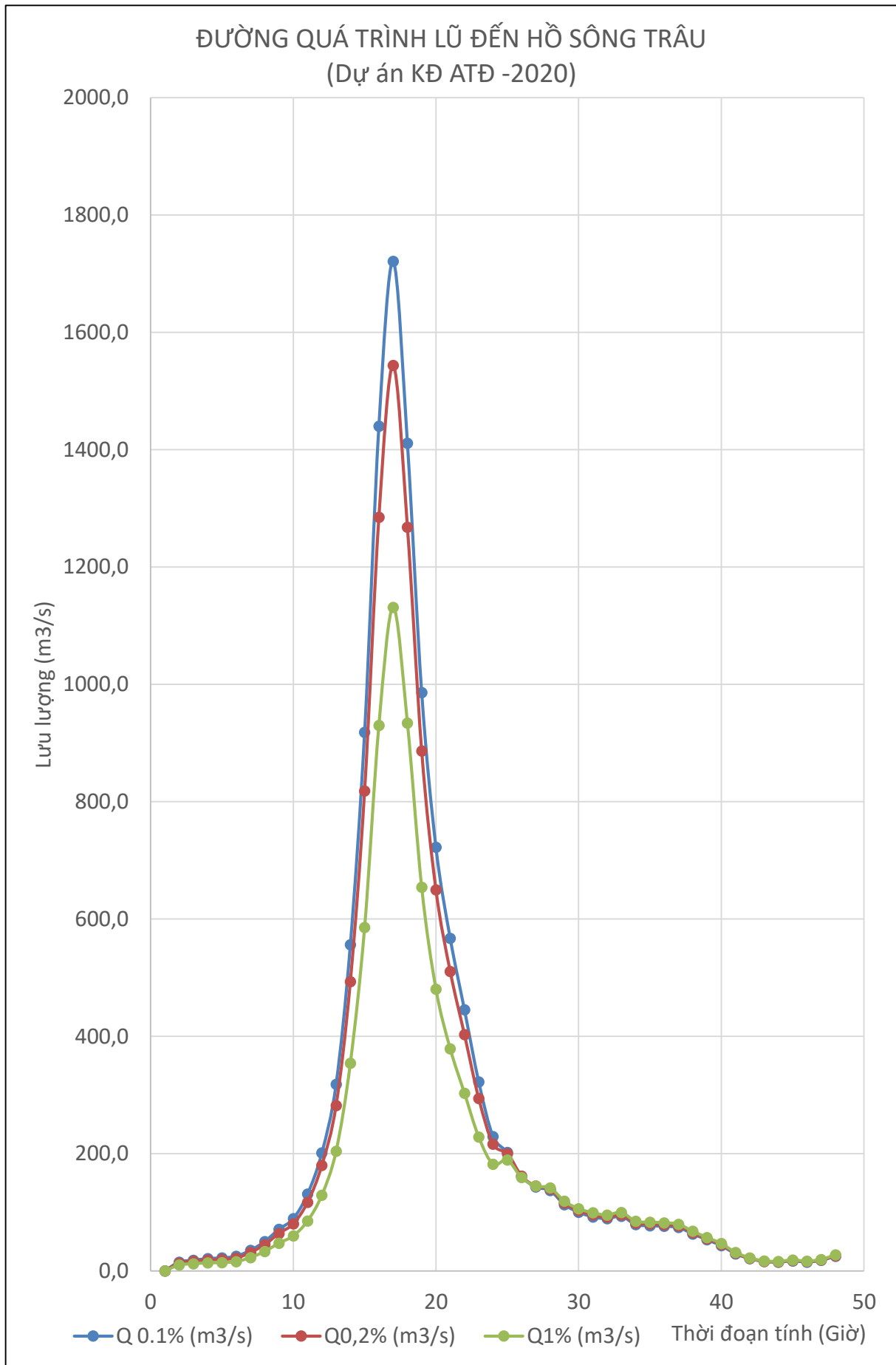
Hình PL 6.3: Hình vẽ quá trình lũ đến hồ Sông Trâu
